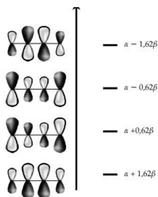
Figure 13. Diagramme des orbitales moléculaire du butadiène.
